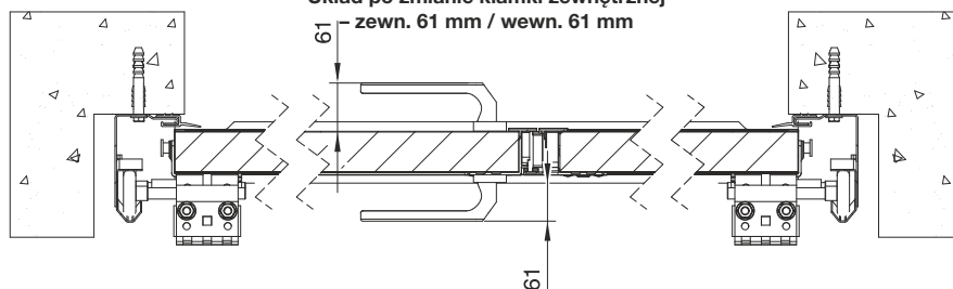
Układ po zmianie klamki zewnętrznej - zewn. 61 mm / wewn. 61 mm
