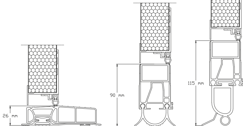
Próg 26 mm + uszczelka (bramy garażowe i przemysłowe)
