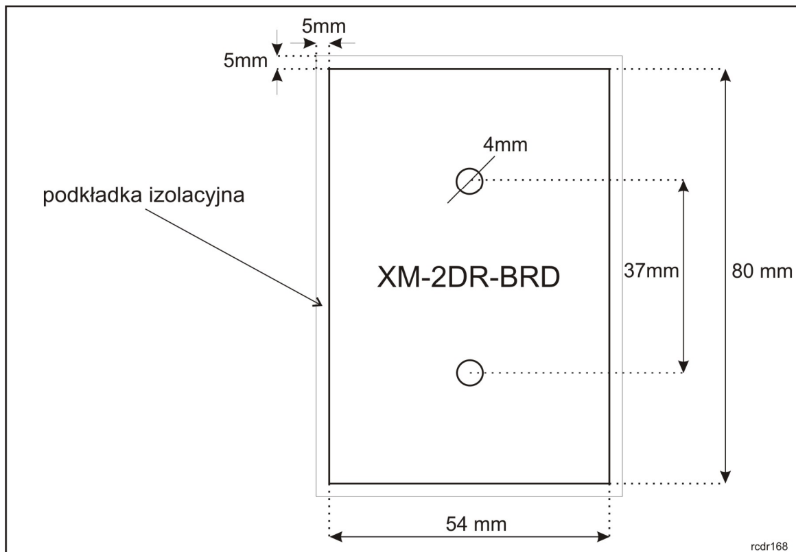
Rys. 3 Rozmieszczenie otworów montażowych modułu XM-2DR-BRD
