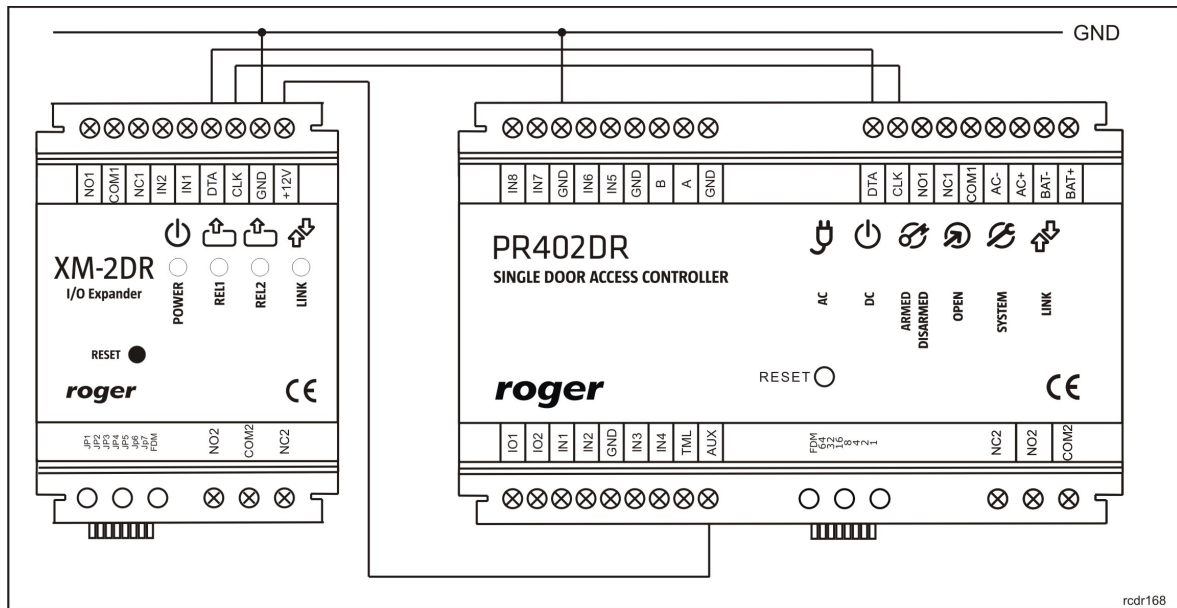
Rys. 2 Podłączenie moduły XM-2DR do kontrolera PR402DR
