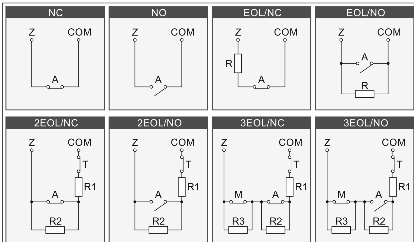
Rys. 4. Sposoby podłączania czujek do wejść. Wyjścia czujki oznaczone są literami: A - alarmowe, T – sabotażowe, M – antymaskingu. R=R_1+R_2 .
