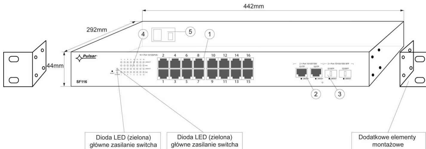
Rys. 2 Widok switch'a.
