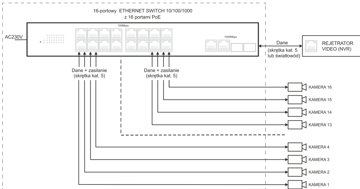
Rys. 1 Schemat blokowy.
