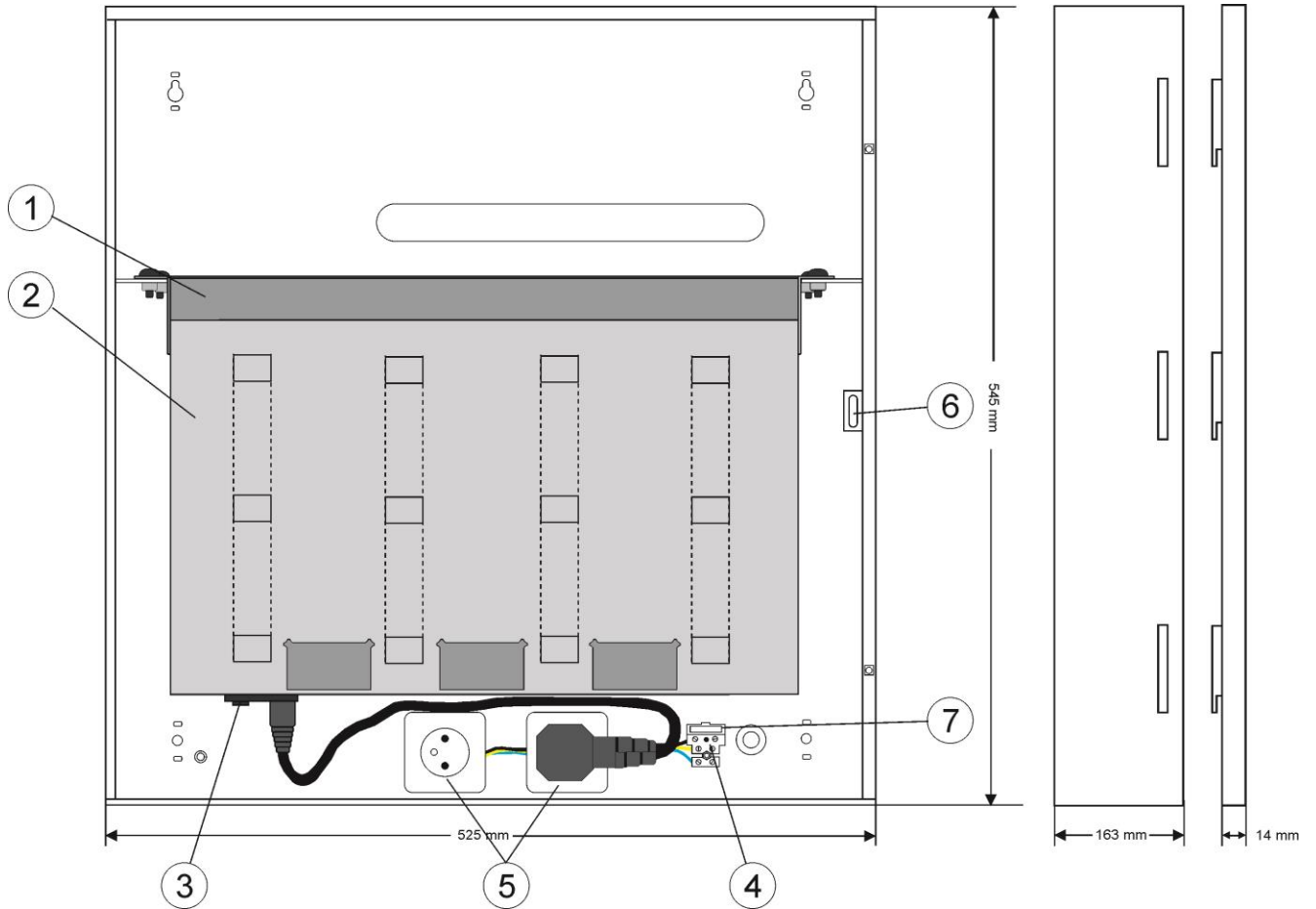
Rys. 2. Widok obudowy.
