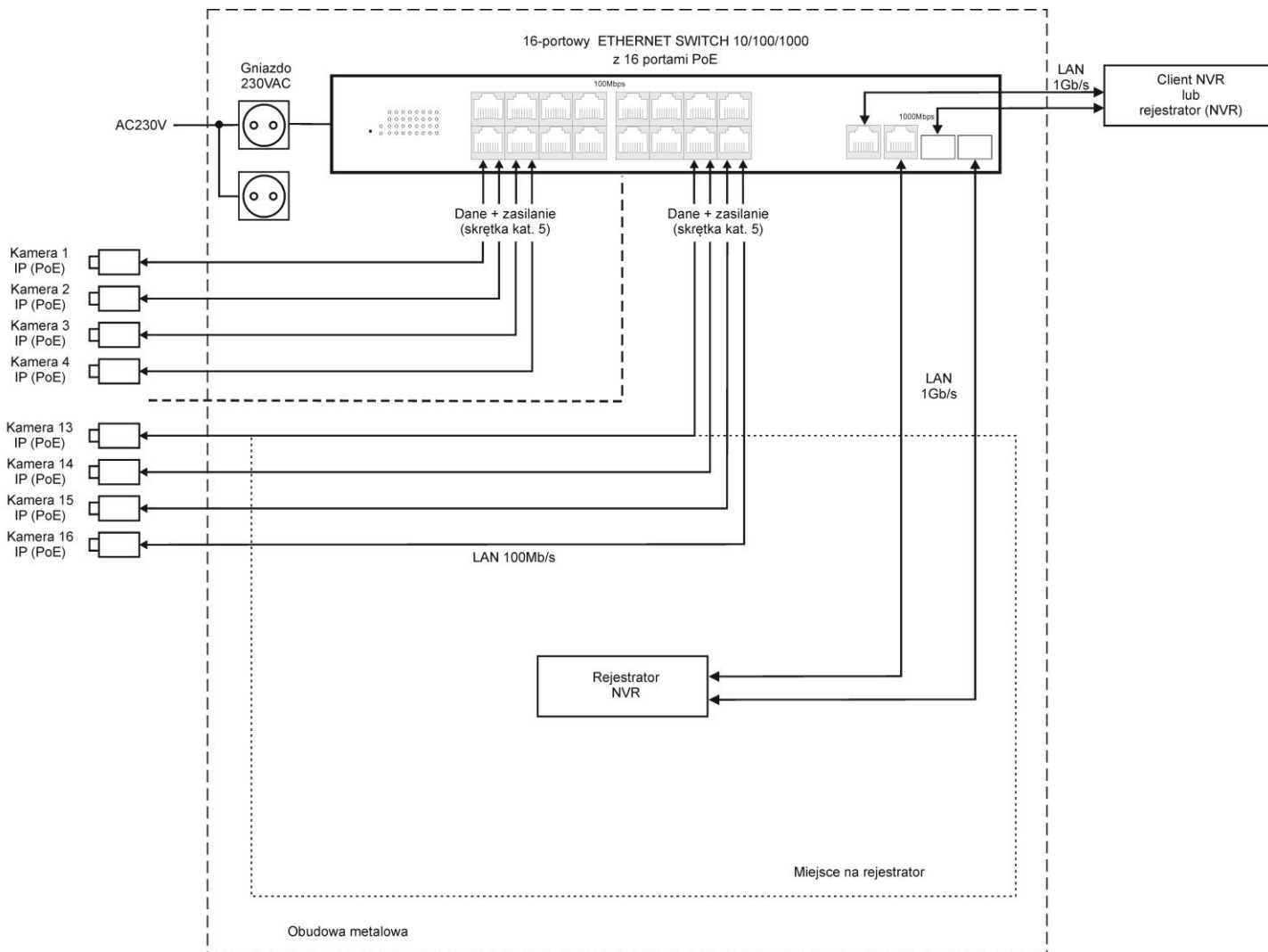
Rys. 1 Schemat blokowy.
