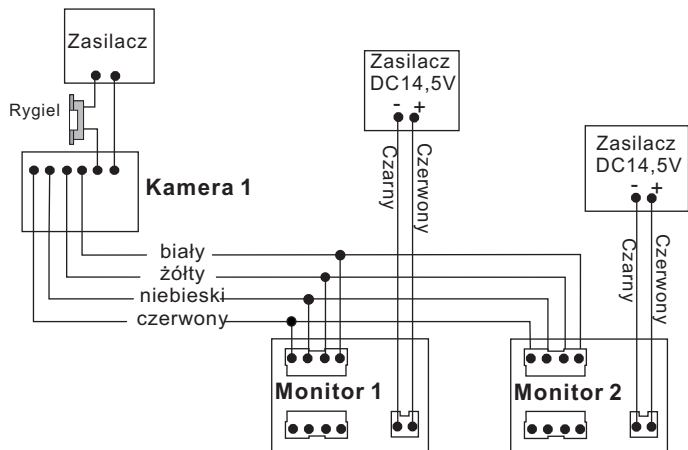
1 kamera + 2 monitory
