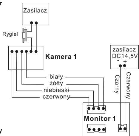
1 kamera + 1 monitor
