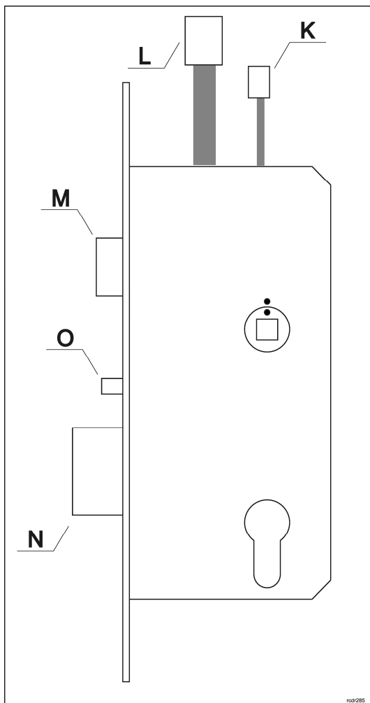
Rys. 6. Zamek wpuszczany
