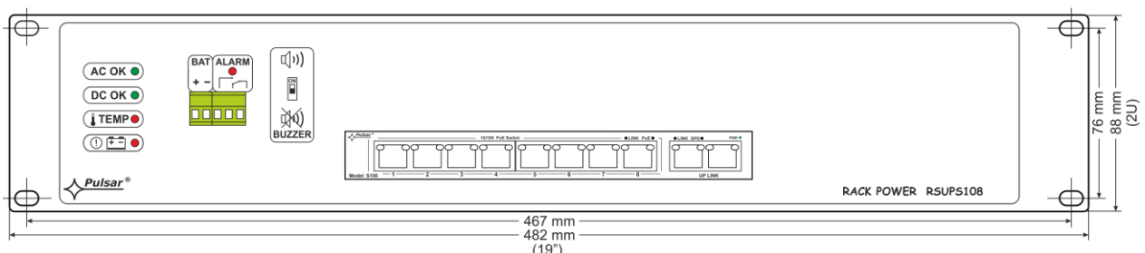
Rys.4. Widok zasilacza.
