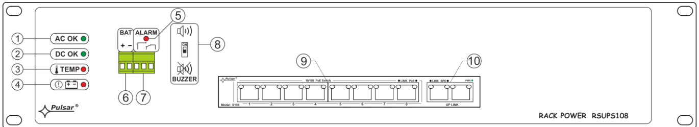
Rys. 2. Panel czołowy zasilacza.
