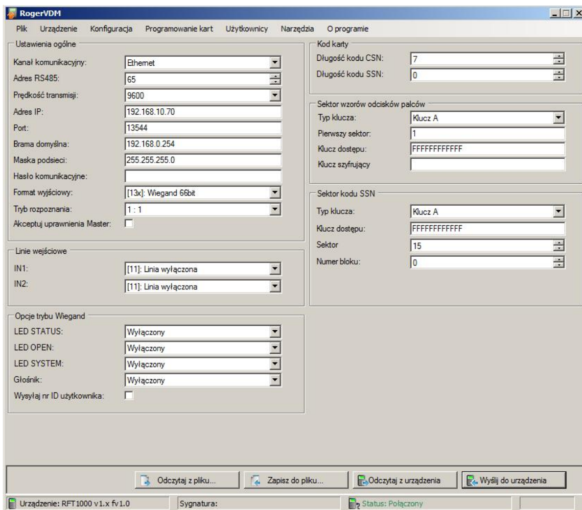
Rys. 5 Okno konfiguracji czytnika RFT1000 w programie RogerVDM
