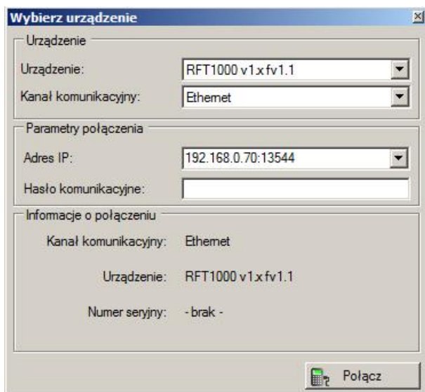
Rys. 4 Okno programu RogerVDM do nawiązania połączenia z czytnikiem
