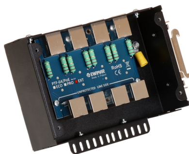
Przykład montażu modułu w obudowie
