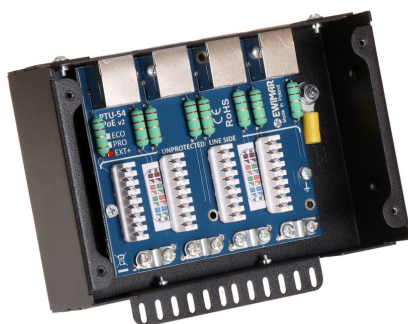
Przykład montażu modułu w obudowie
