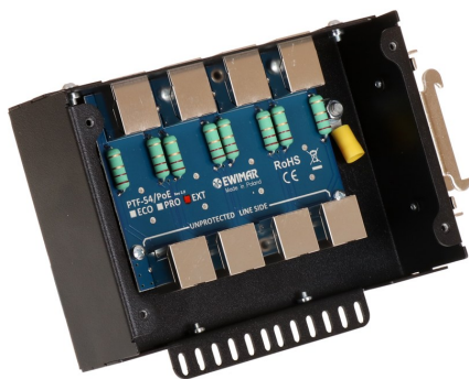
Przykład montażu modułu w obudowie
