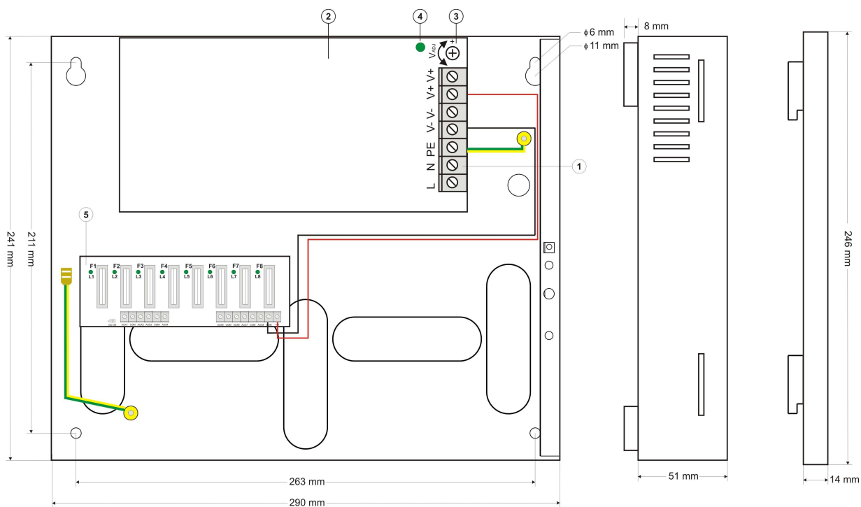
Rys.3. Widok zasilacza.
