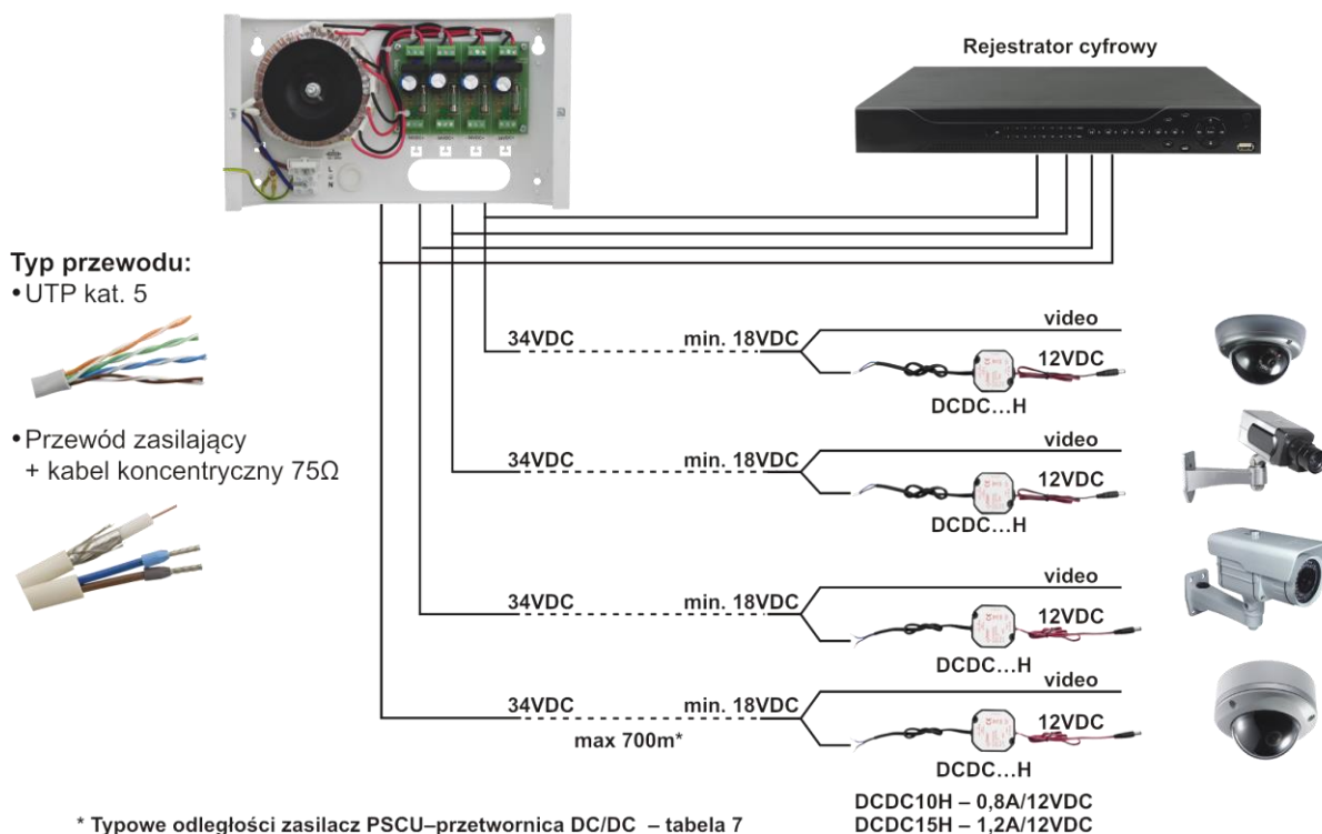
Rys.4. Instalacja zasilacza PSCU04344SEP.
