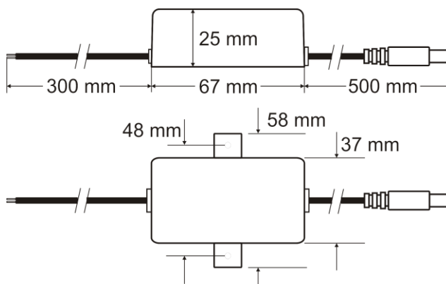
Rys.1. Widok mechaniczny zasilacza.
