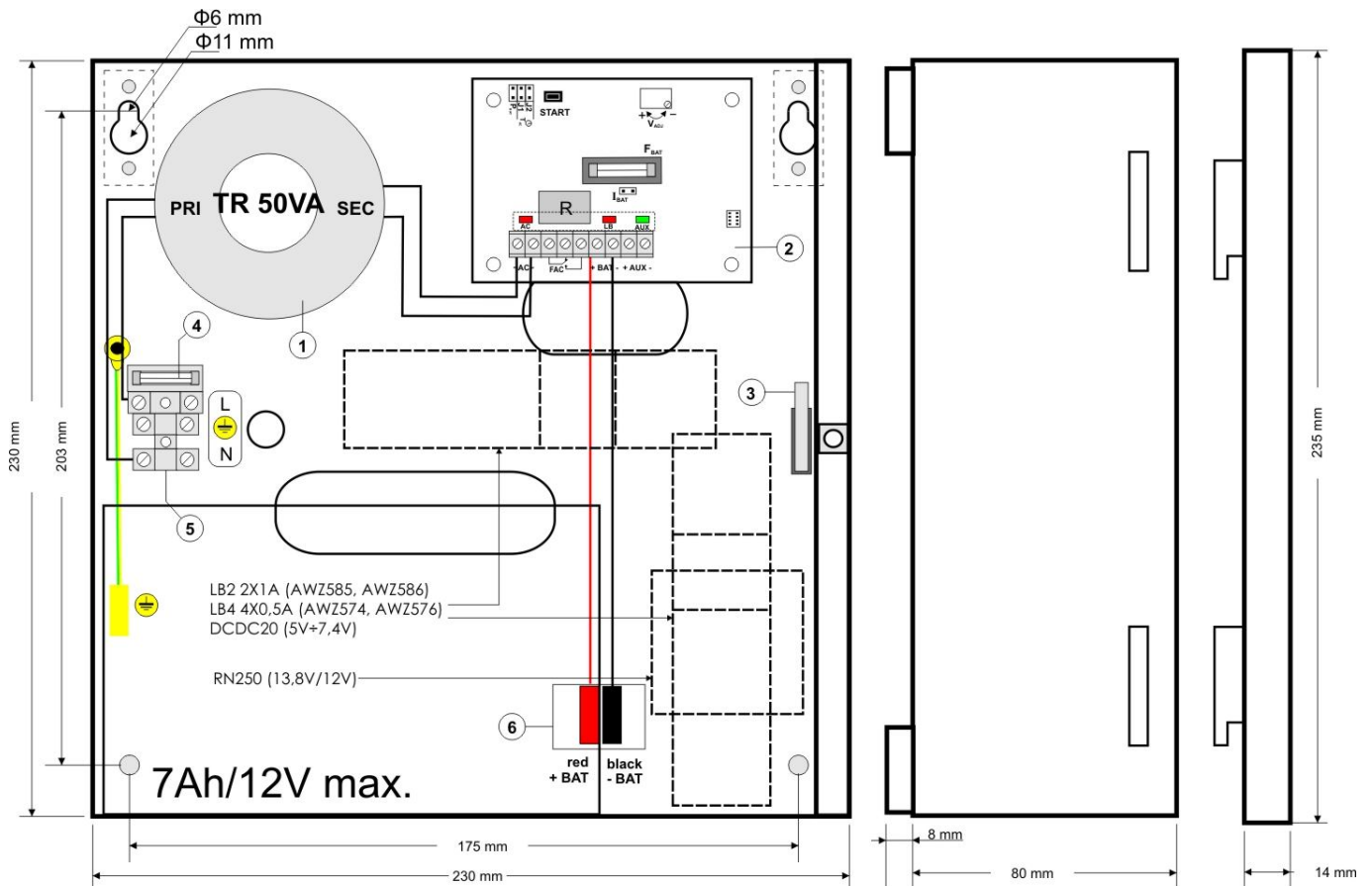
Rys.3. Widok zasilacza.
