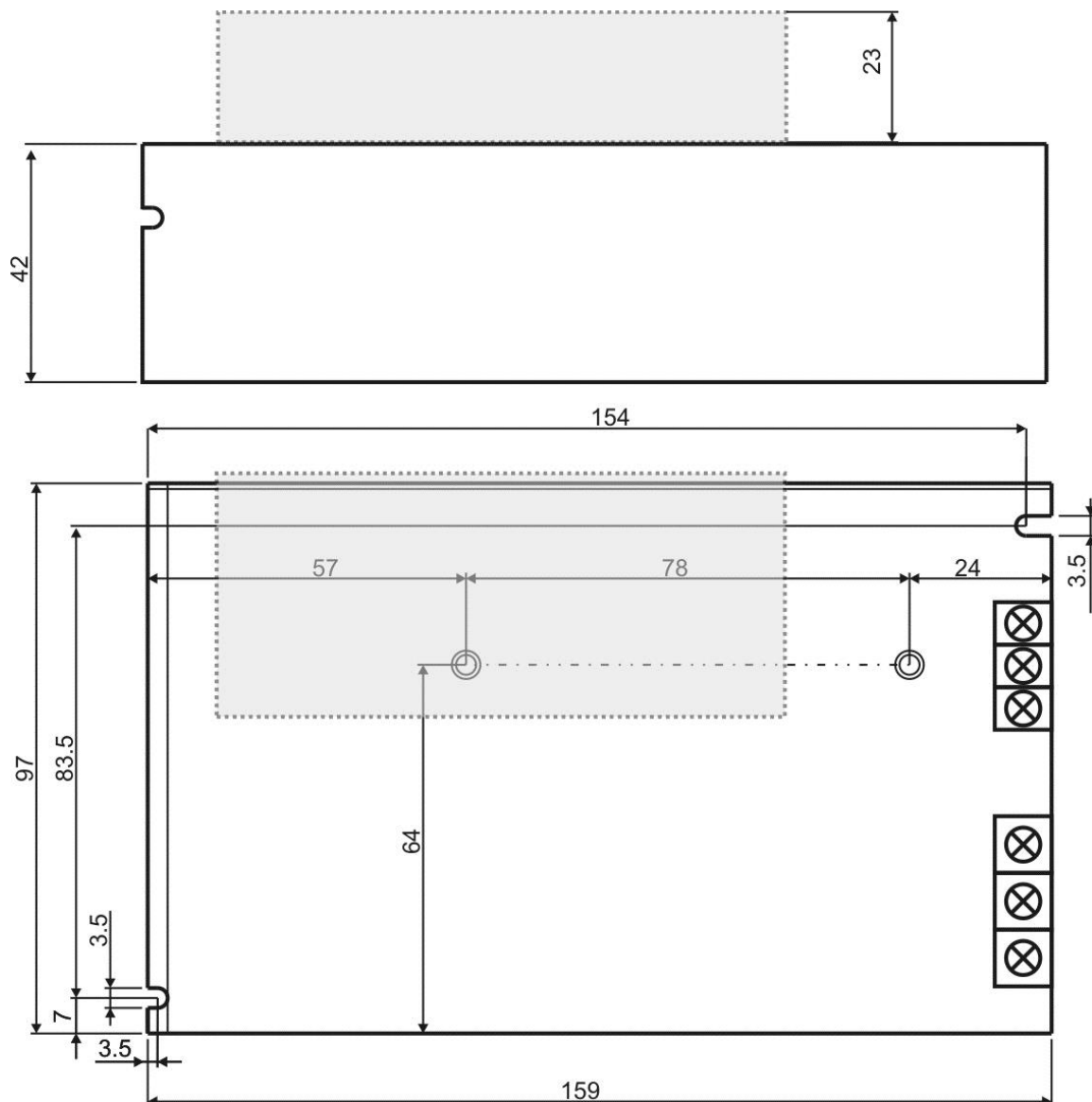
Rysunek 3. Widok mechaniczny zasilacza.
