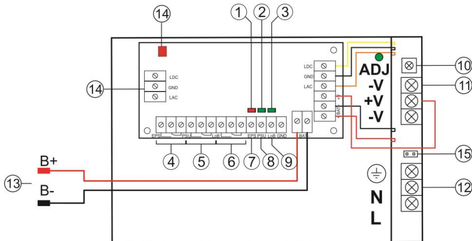
Rys. 2. Widok zasilacza.
