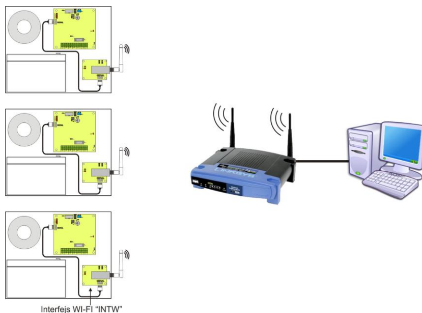
Rys. 15. Komunikacja Wi-Fi z wykorzystaniem interfejsu Wi-Fi „INTW”.
