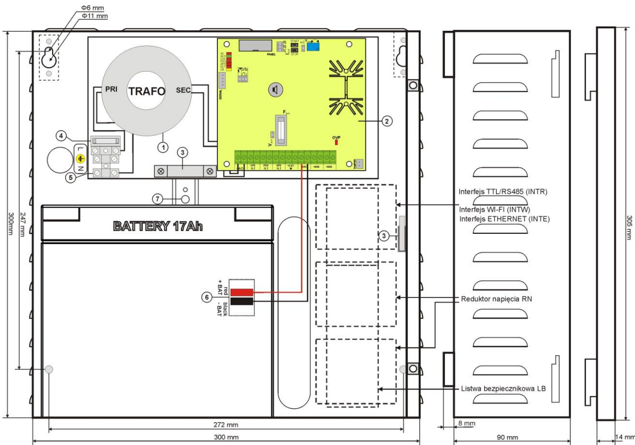
Rys.3. Widok zasilacza.
