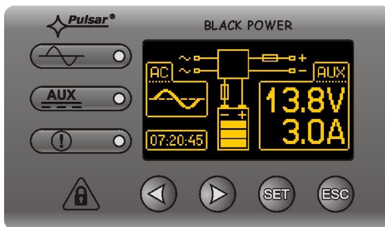
Rys. 5. Panel kontrolny.
