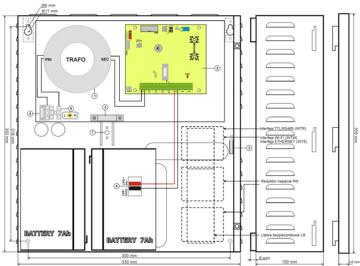
Rys.3. Widok zasilacza.
