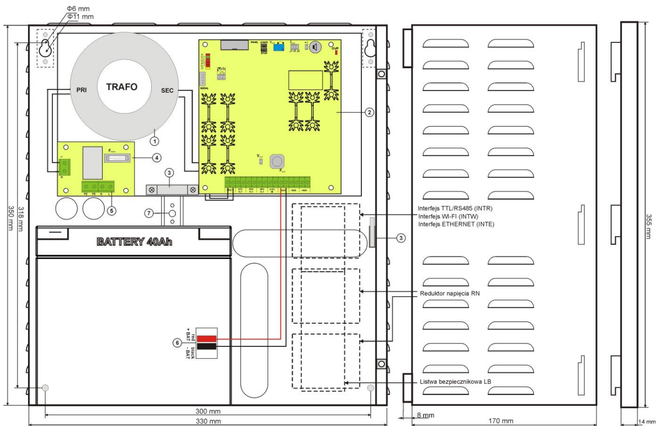
Rys.3. Widok zasilacza.
