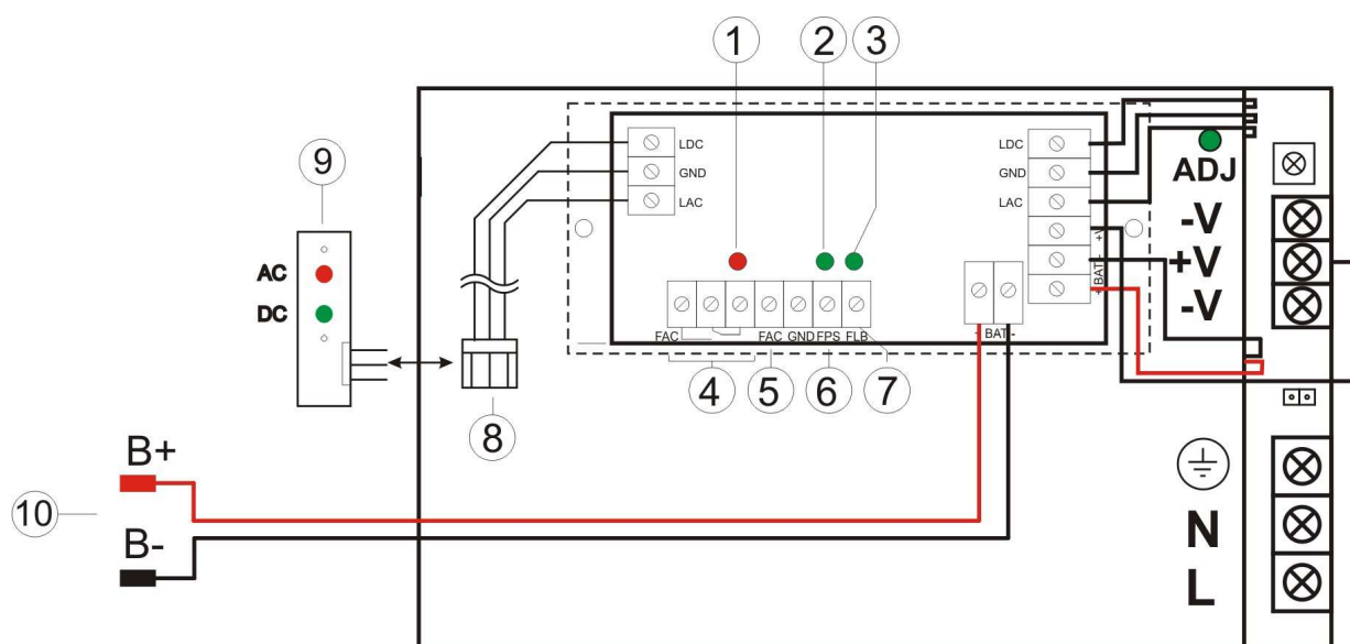
Rysunek. 3. Widok zasilacza z modułem MPSB12.
