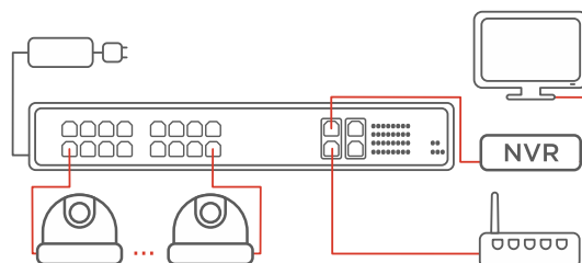
Schemat przykładowego podłączenia PIX-POE16AT-2GE-2SFP
