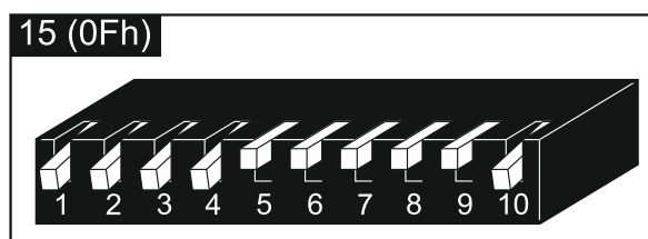
Rys. 11. Sposób ustawienia przełączników DIP-switch w ekspanderze INT-ORS.
