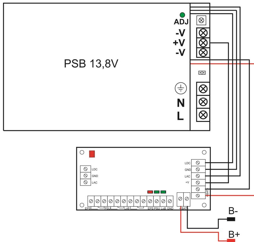
Rys.2 Schemat podłączenia modułu do zasilacza PSB.
