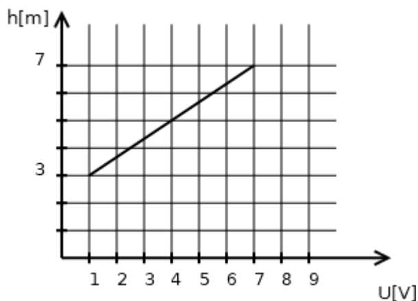
Charakterystyka czujnika.
