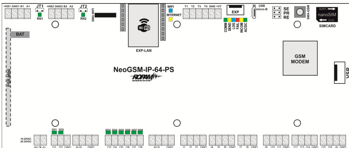
Widok: NeoGSM-IP-64-PS PCB.
