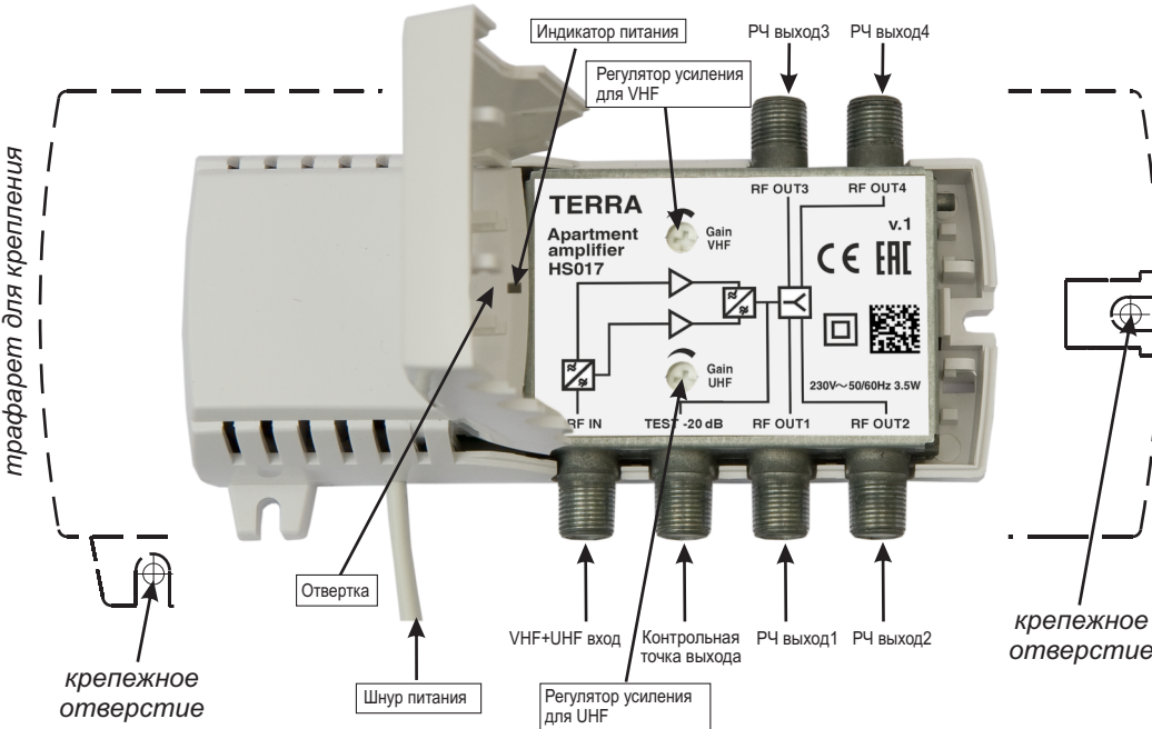
Рис.1. Внешний вид усилителя и органы управления
