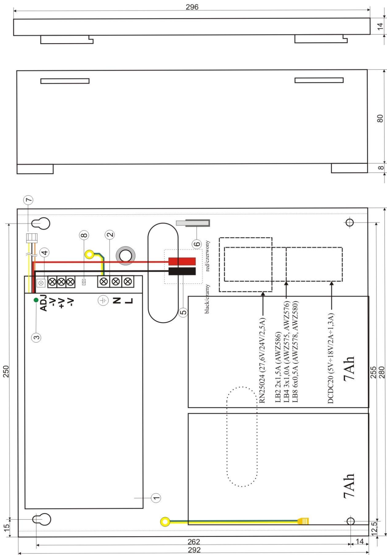
Rys.2. Widok zasilacza.
