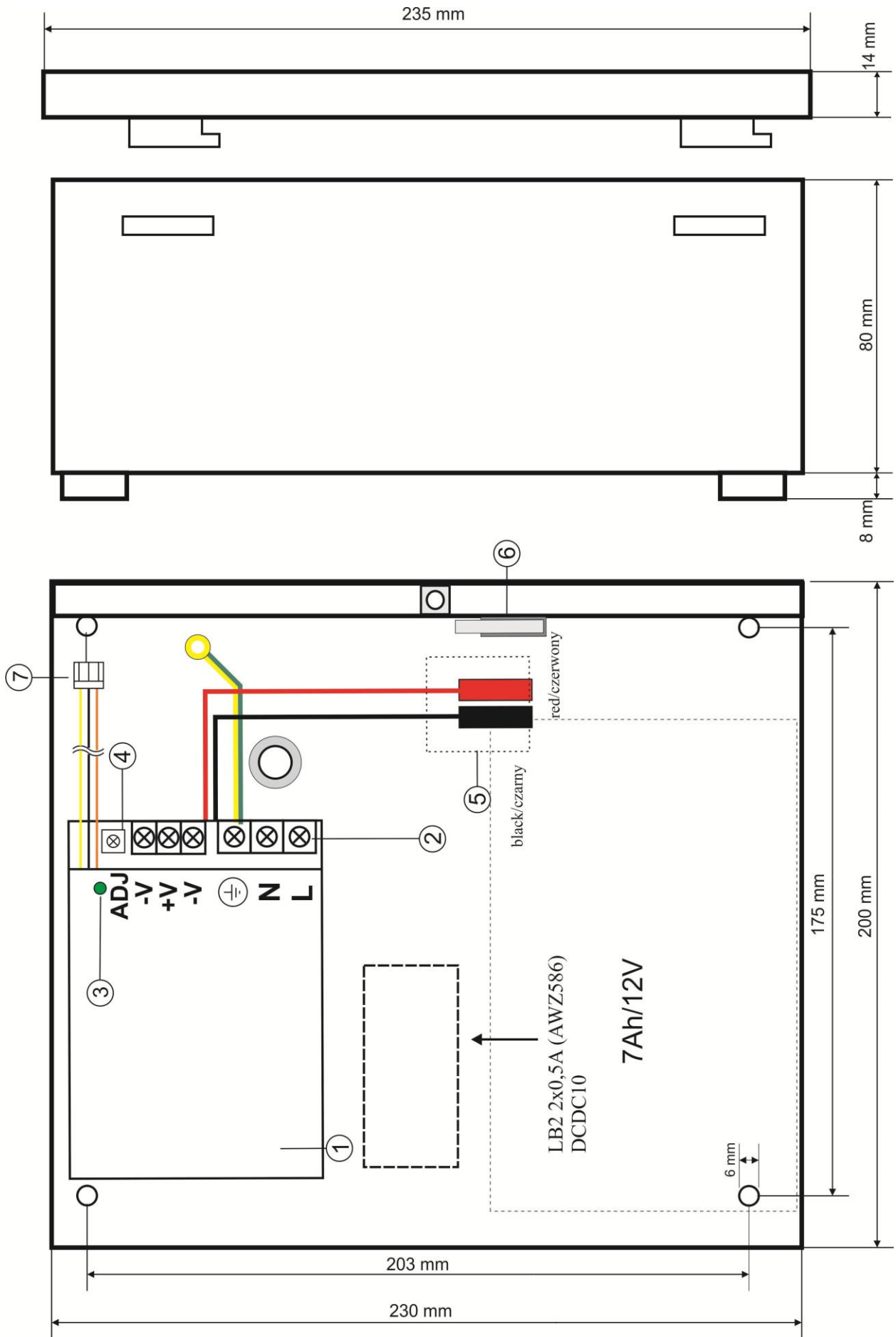
Rys.2. Widok zasilacza.
