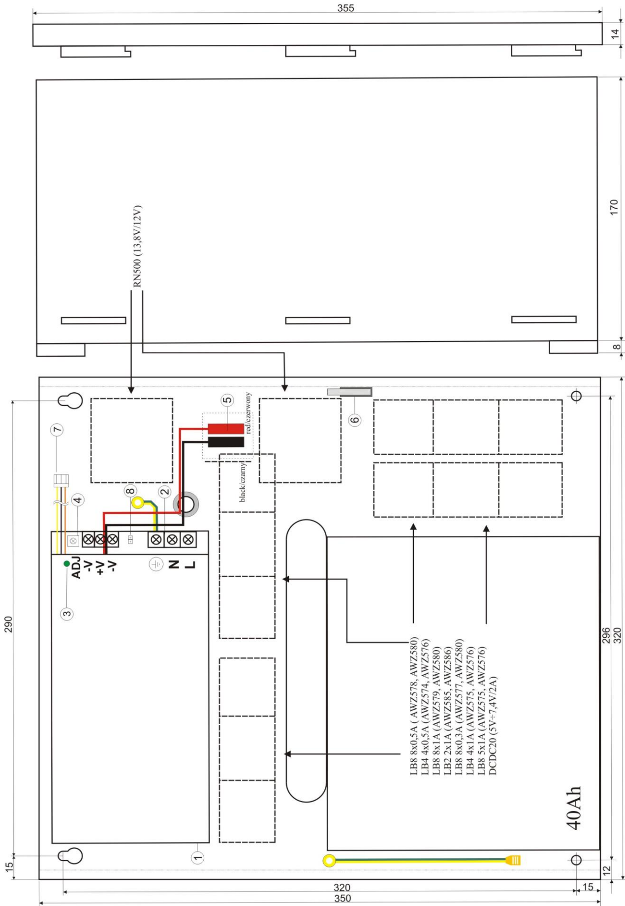
Rys.2. Widok zasilacza.
