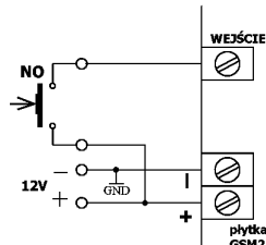
A. Sterowanie przez podanie +12V Ustawić poziom aktywny H
