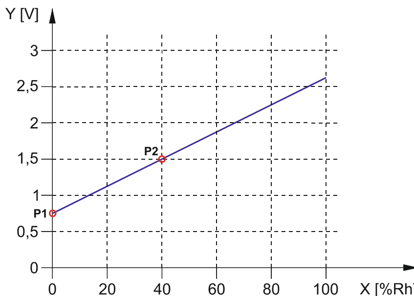
Rys. 22. Przykładowa charakterystyka liniowa czujnika wilgotności powietrza, gdzie: X – wilgotność względna [%Rh], Y – napięcie na wyjściu czujnika [V].
