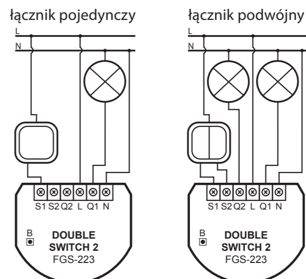
Schematy podłączenia - Double Switch 2
