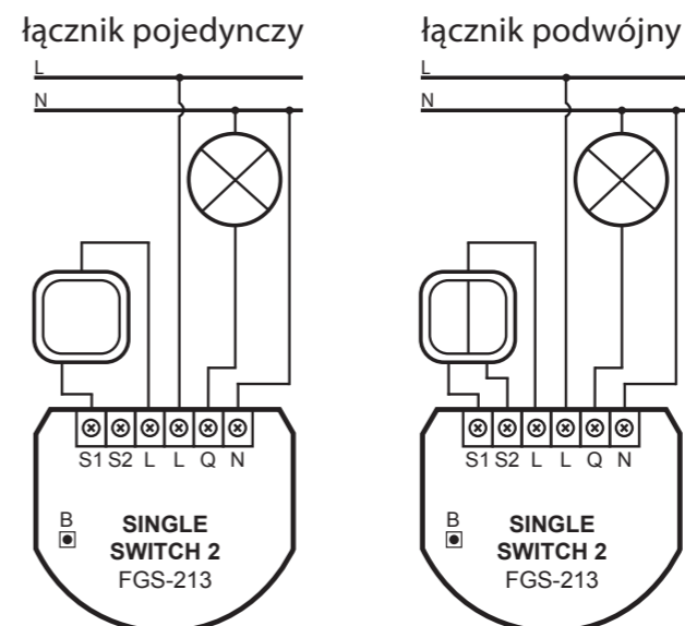
Schematy podłączenia - Single Switch 2
