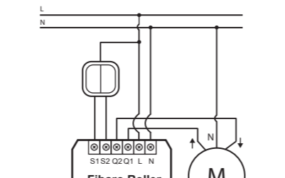
Rys. 1 Schemat elektryczny podłączenia Fibaro Roller Shutter'a
