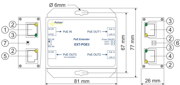
Rys.1. Rysunek urządzenia.
