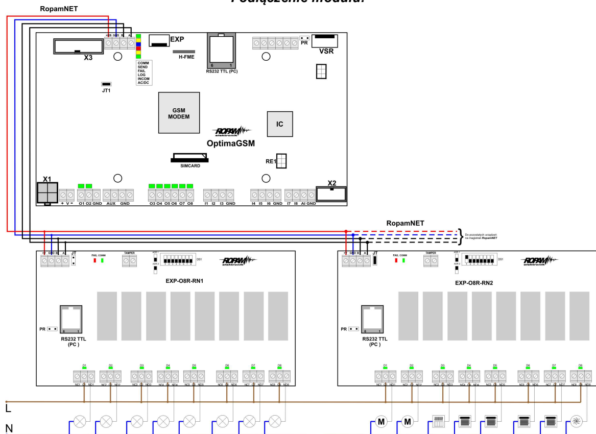
Podłączenie modułu:
