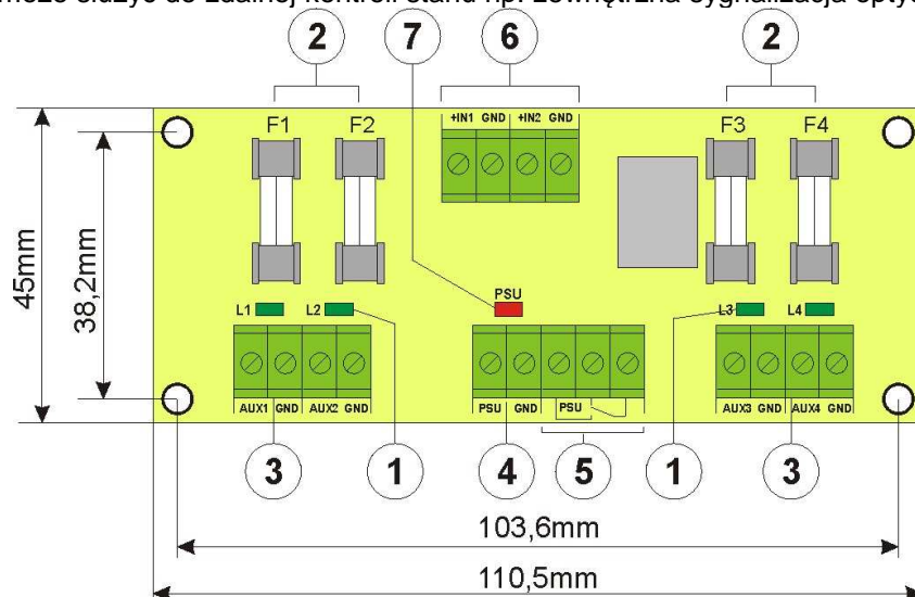
Rys.1. Widok modułu.
