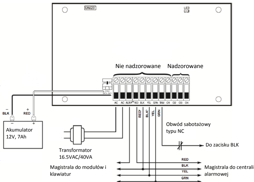
Rysunek 2-6 Moduł rozszerzeń wyjść programowalnych HSM2208
