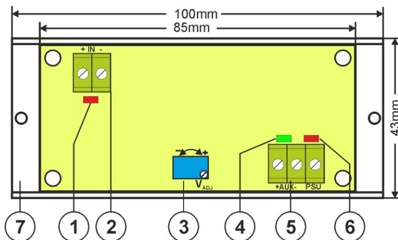
Rys.2. Widok modułu przetwornicy.
