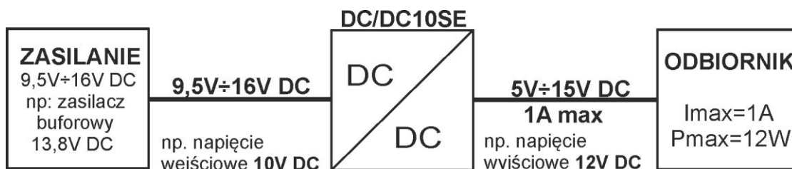
Regulacja napięcia wyjściowego przetwornicy 5V÷15V DC, 1A max.
