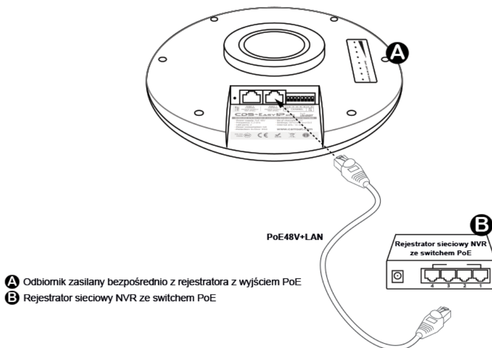
Podłączenie i zasilanie odbiornika z rejestratora NVR ze switchem PoE
