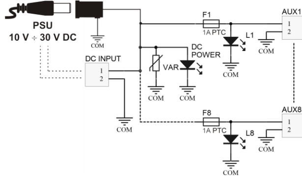
Rys.2. Schemat blokowy.
