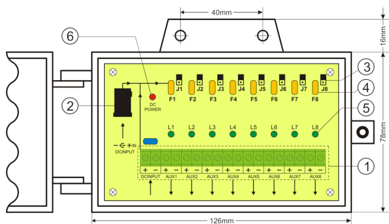
Rys.1. Rysunek modułu.
