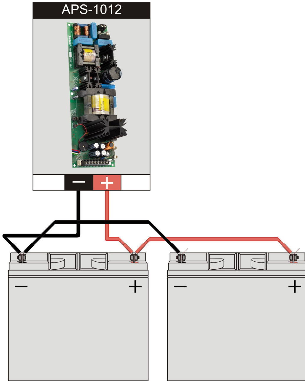
Rys. 4. Równoległe połączenie dwóch akumulatorów. Połączenie można wykonać przy pomocy kabli dostępnych w zestawie z urządzeniem.
