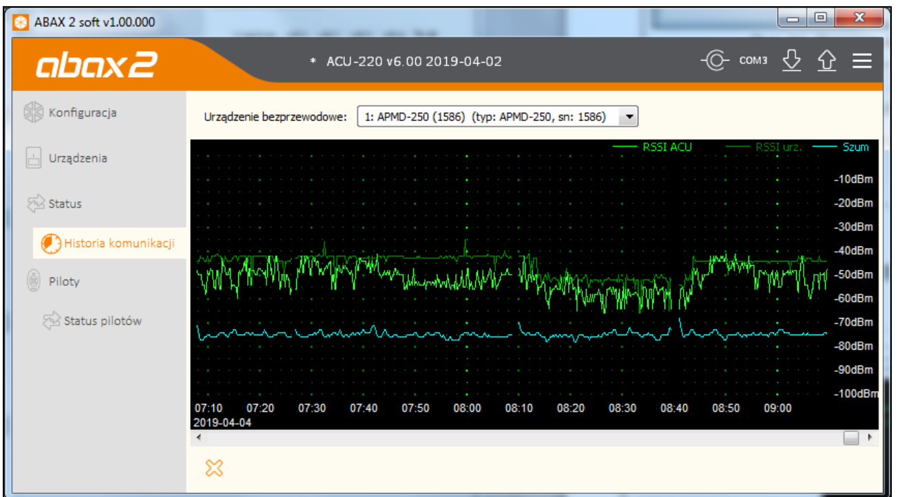
Rys. 14. Program ABAX 2 Soft: zakładka „Historia komunikacji”.
