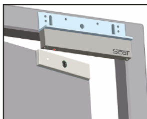
Montaż z uchwytem BK-600WL
