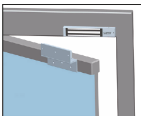
Montaż z uchwytem BK-600WZL
