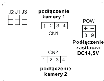
Wymiary: 160x120x42mm
