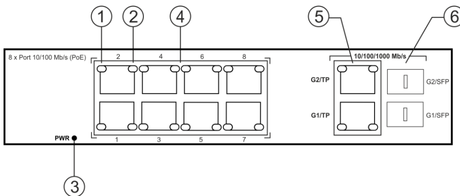
Rys.2. Widok Switch'a.
