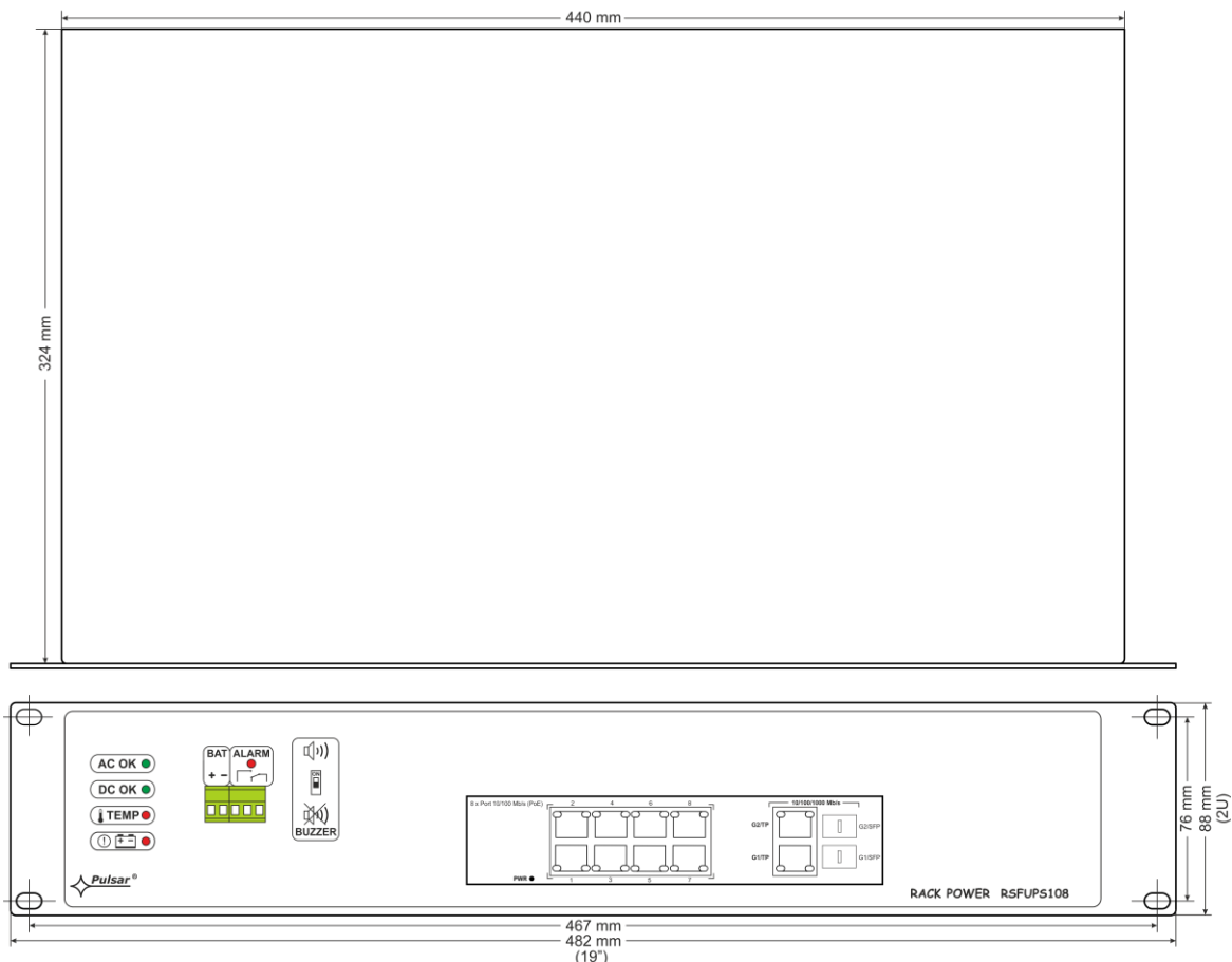
Rys.5. Widok zasilacza.
