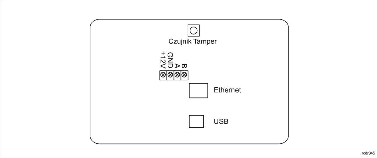
Rys. 3 Wewnętrzna strona panelu przedniego RCC512
