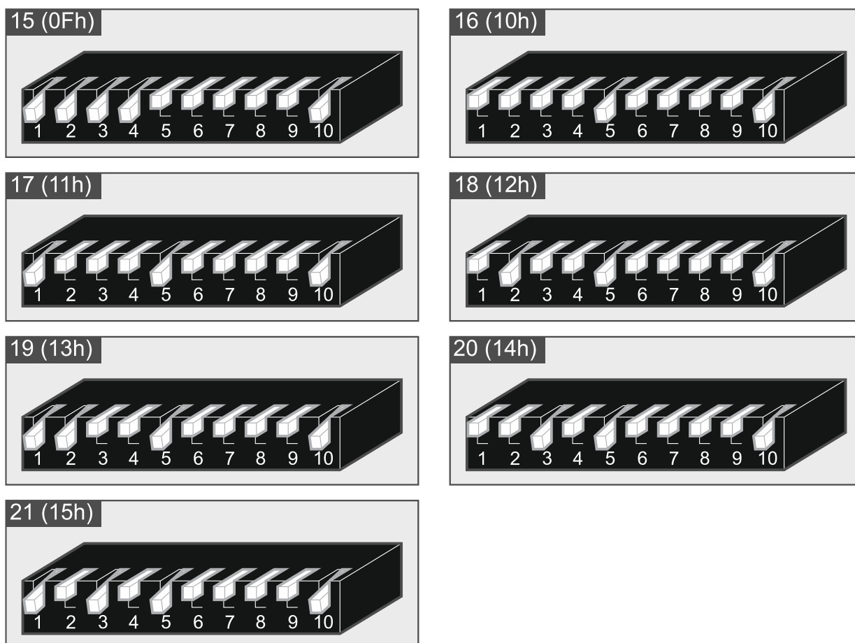
Rys. 15. Ustawienie przełączników DIP-switch w ekspanderze INT-ORS.
