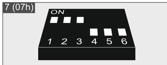
Rys. 10. Ustawienie przełączników DIP-switch w ekspanderze INT-RX-S.
