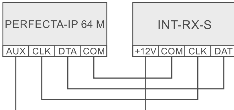
Rys. 9. Podłączenie ekspandera INT-RX-S do centrali.
