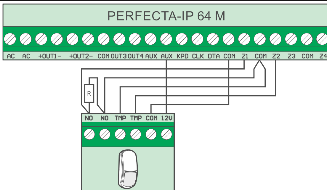
Rys. 22. Przykład podłączenia czujki NO w konfiguracji EOL.
