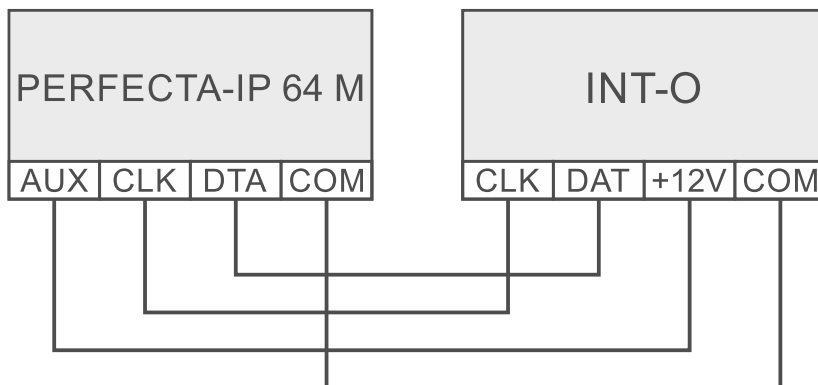
Rys. 13. Podłączenie ekspandera INT-O do centrali.
