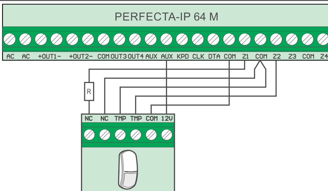
Rys. 21. Przykład podłączenia czujki NC w konfiguracji EOL.
