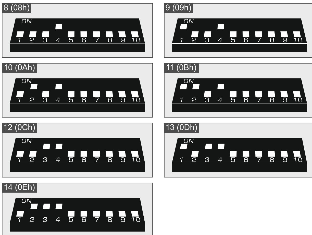
Rys. 12. Ustawienie przełączników DIP-switch w ekspanderze INT-E.
