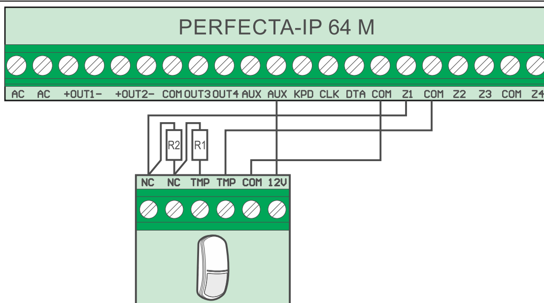
Rys. 23. Przykład podłączenia czujki NC w konfiguracji 2EOL (czujkę NO podłącz identycznie).
