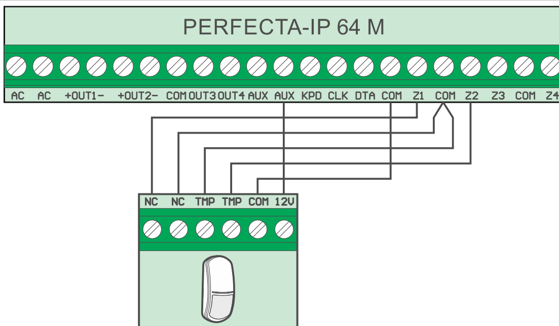
Rys. 20. Przykład podłączenia czujki NC (czujkę NO podłącz identycznie).
