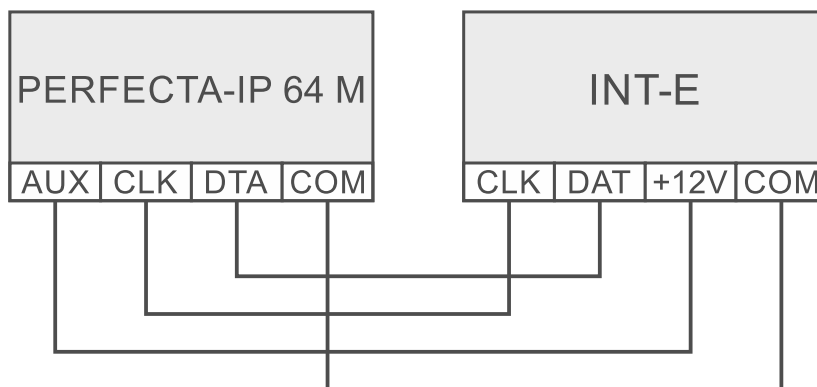
Rys. 11. Podłączenie ekspandera INT-E do centrali.
