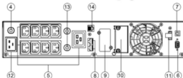
OLS3000ERT/ERT(XL)2U
