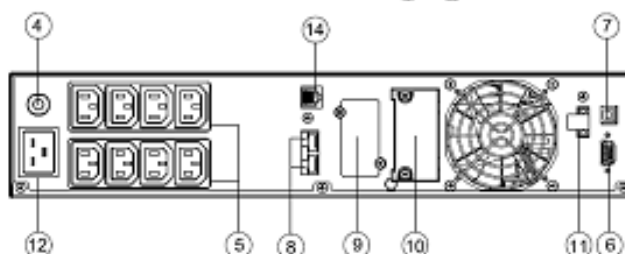
OLS2000ERT(XL)2U
