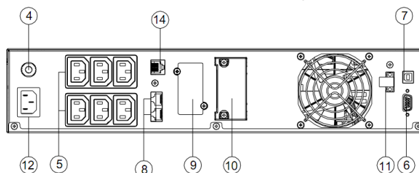
OLS1000ERT(XL)2U, OLS1500ERT(XL)2U
